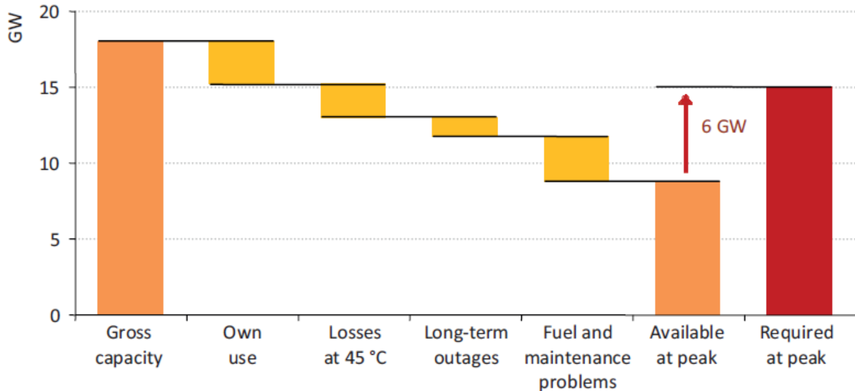
イラクの発電施設容量と実際のピーク発電量のギャップ発生分布
