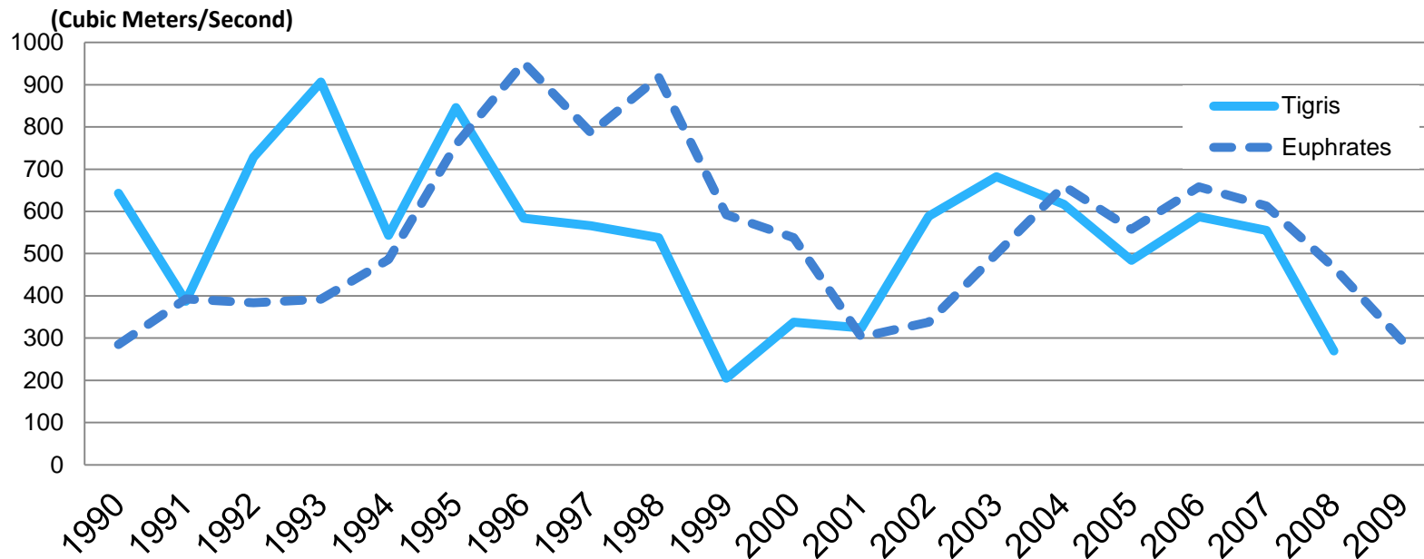
チグリス川・ユーフラテス川の平均流量の推移
